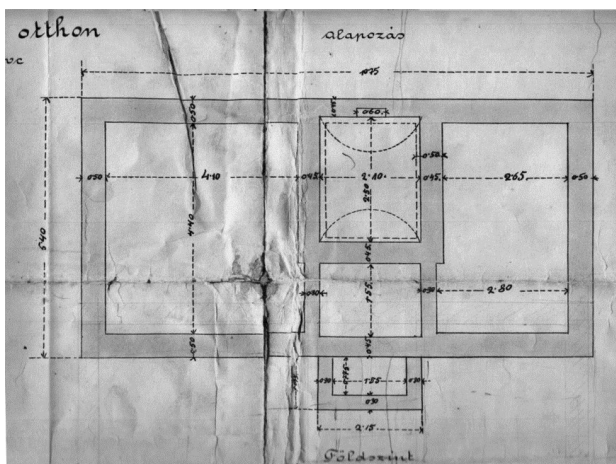
Benedek Dezső tervező: Kétszobás títusterv (Forrás: Tóth Krisztina építésmérnök)
