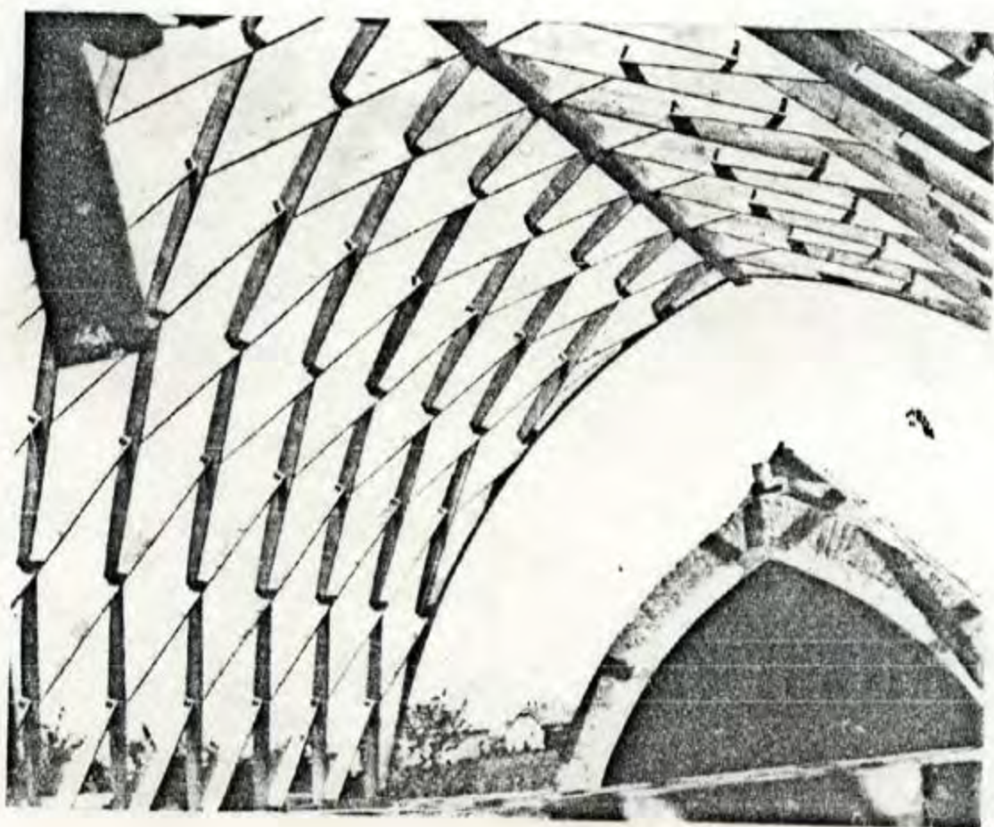
A TEMPLOM -OIKOSZ.-RENDSZERŰ FEDELSZÉKE ÁLLÍTÁS KÖZBEN
